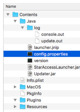
Рис.8. Вміст папки Java.
